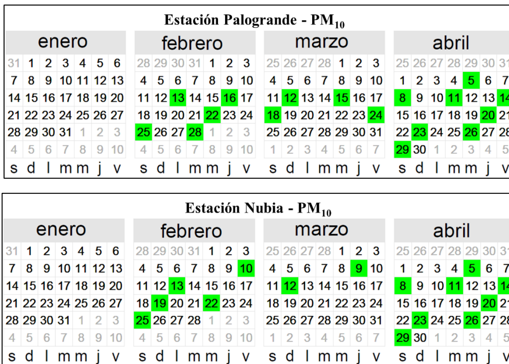
Figura 4. Índice de Calidad del Aire (ICA) para PM 10 durante primer cuatrimestre de 2017.
