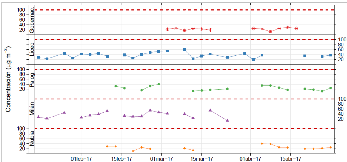
Figura 3. Evolución temporal de concentraciones diarias de PM 10 entre enero y abril de 2017. El límite máximo permisible diario (100 µg/m 3 ) según la Resolución 610 de 2010 se muestra en la línea punteada roja.
