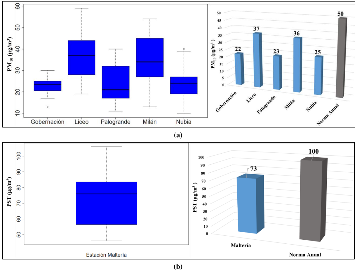
Figura 2. Diagrama de cajas y concentración promedio del primer cuatrimestre del año comparada con norma anual en las estaciones de monitoreo. a) Concentraciones promedio aritmético PM 10 . b) Concentraciones promedio geométrico PST.
