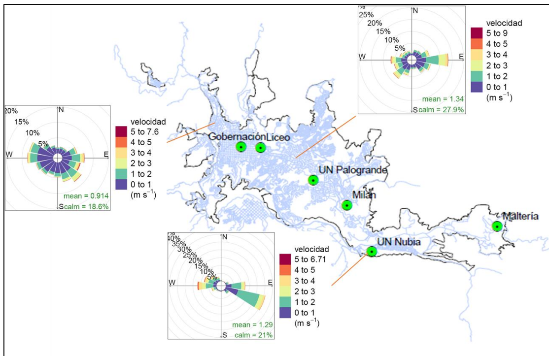
Figura 1. Mapa de Manizales con ubicación de las estaciones de calidad del aire y rosas de viento de estaciones meteorológicas representativas para el periodo enero-abril del 2017.
